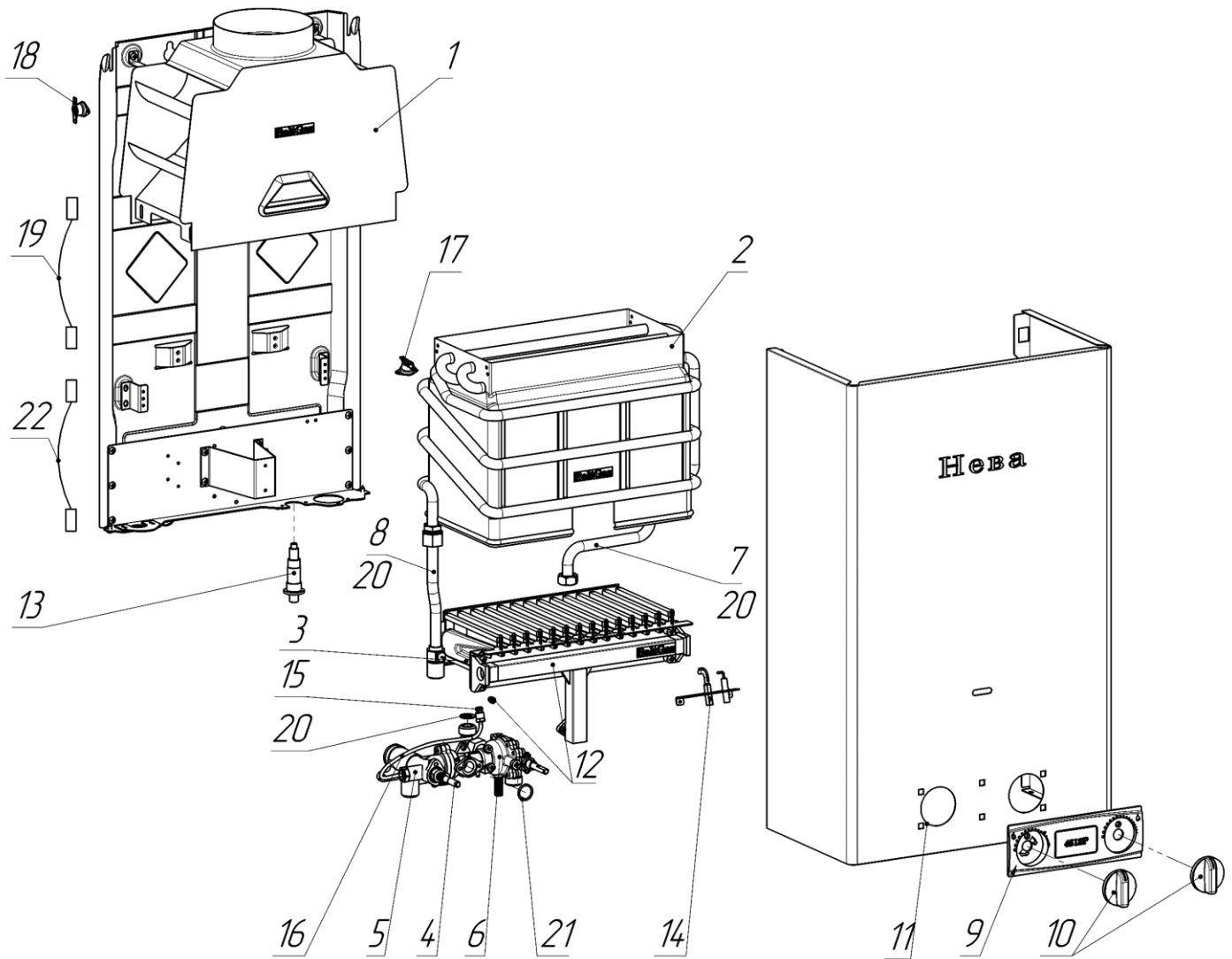
Рисунок 11. Вид аппарата с разнесёнными частями
